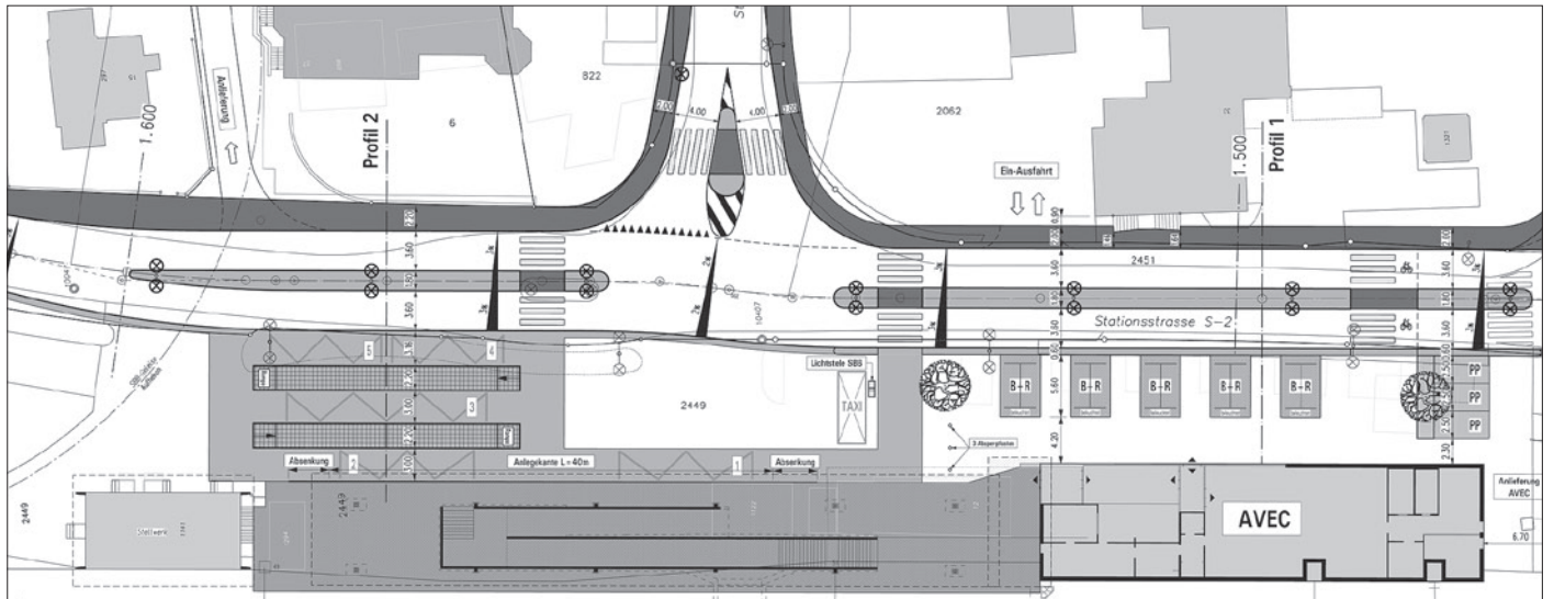
Ausschnitt Situationsplan (Vorprojekt) Bahnhof Bonstetten-Wetzwil. (Grafik zVg)
